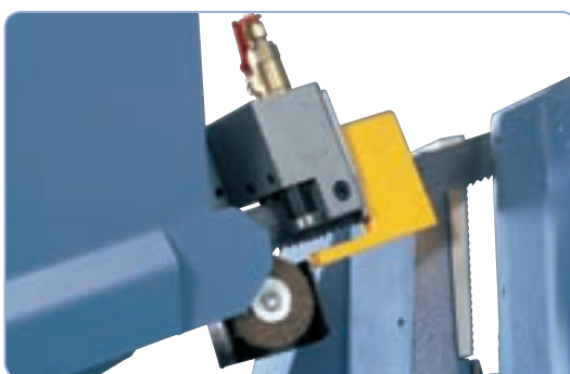
Kuulalaakeroidut teränohjaimet ja lastuharja ideaaliin sahaustuloksiin
