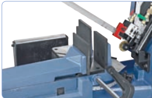
Kiinteä valurauta kappaleenpuristin jossa pikalukitusmekanismi, ihanteellinen toistuviin sahuksiin
