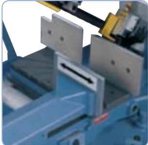
Pikakappaleenkiinnitys voidaan siirtää terän molemmille puolille
