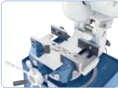
Keskitetty kappaleenkiinnitys sisältää vaakatasossa säädettävät leuat
