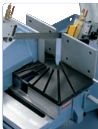
Ruuvipuristinta voi liikuttaa sivuttain
