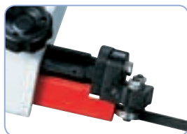
Teränohjaimet laakeroitu ja säädettävissä joka työkappaleelle
