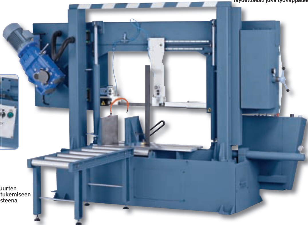
Teänohjaimet voidaan säätää täydellisesti joka työkappaleelle
