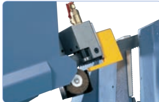
Laakeroidut teränohjaimet ja terähärja takaavat tarkan työtuloksen
