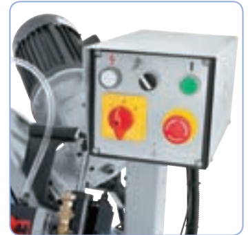
Helppokäyttöiset käyttökytkimet ohjainpaneelissa
