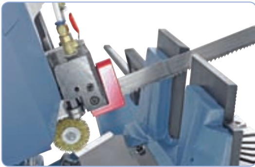
Teränohjaimet laakeroitu ja säädettävissä nopeasti joka työkappaleelle, tämä takaa optimaalisen sahaustuloksen
