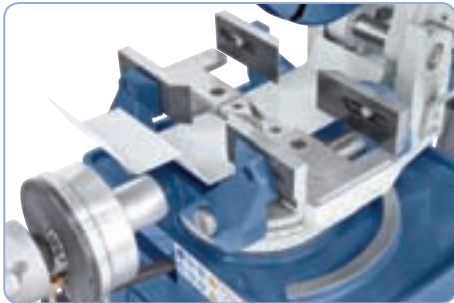
Pneumaattinen kappaleen pikakiinnitys lyhentää asennusaikoja
