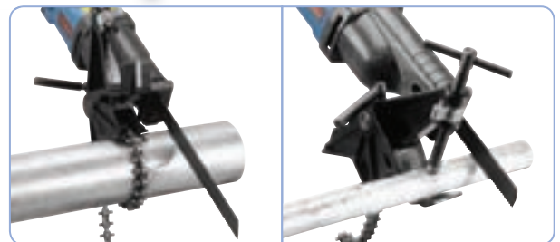
Lisävarusteena saatavilla: 2 in 1 puristin – voidaan käyttää ketjulla teräsputkia sahattaessa 1" – 6" tai pikavapautus putkipuristin missä mahdollisuus kulmaan sahattaessa 90°
